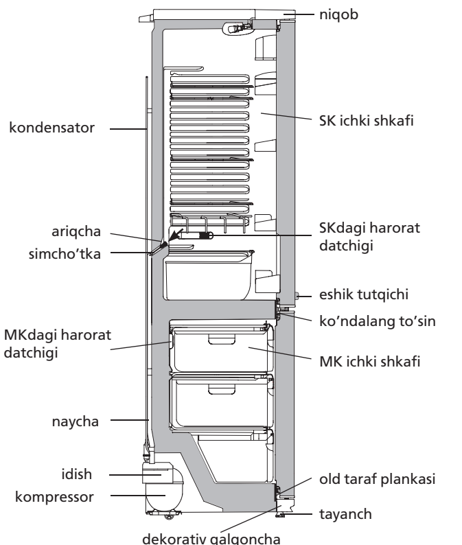
7 rasmi — SKdan erigan suvni tushirish chizmasi
